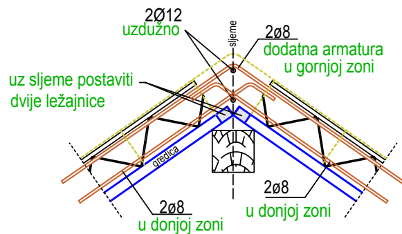
detalj sjemena 1
