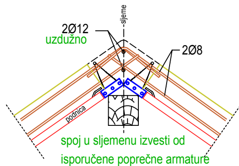
detalj sjemena 2
