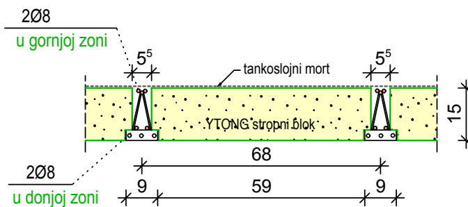
poprečni presjek Ytong stropa kroz grebnice
