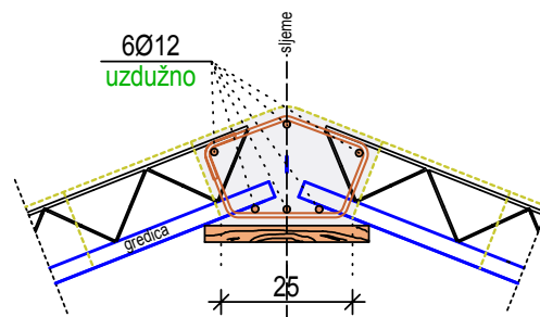
detalj sjemena 3
